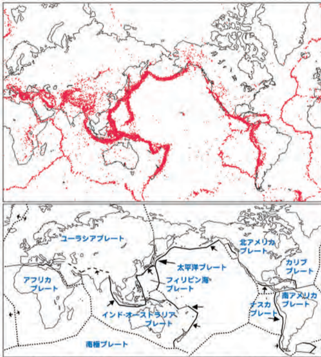
【図1】世界の地震の震央分布とプレートの分布。上図は1990年から2000年までに起こったM(マグニチュード)4以上、深さ50kmより浅い地震の震央を示している(気象庁ホームページhttp://www.jma.go.jp/jma/kishou/now/whitep/2-1.htmlより転載)
