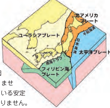
【図2】日本列島周辺のプレートの配置
