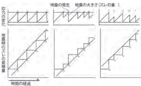
図7-1 地震が繰り返し発生する場合の③モデル (Shimazaki and Nakata, 1980による)
