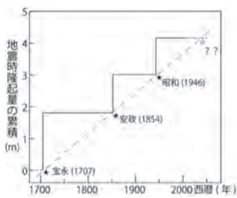
図7-2 南海地震による高知県室戸市室津港における隆起量 (Shimazaki and Nakata, 1980による) と地震の発生間隔の関係
