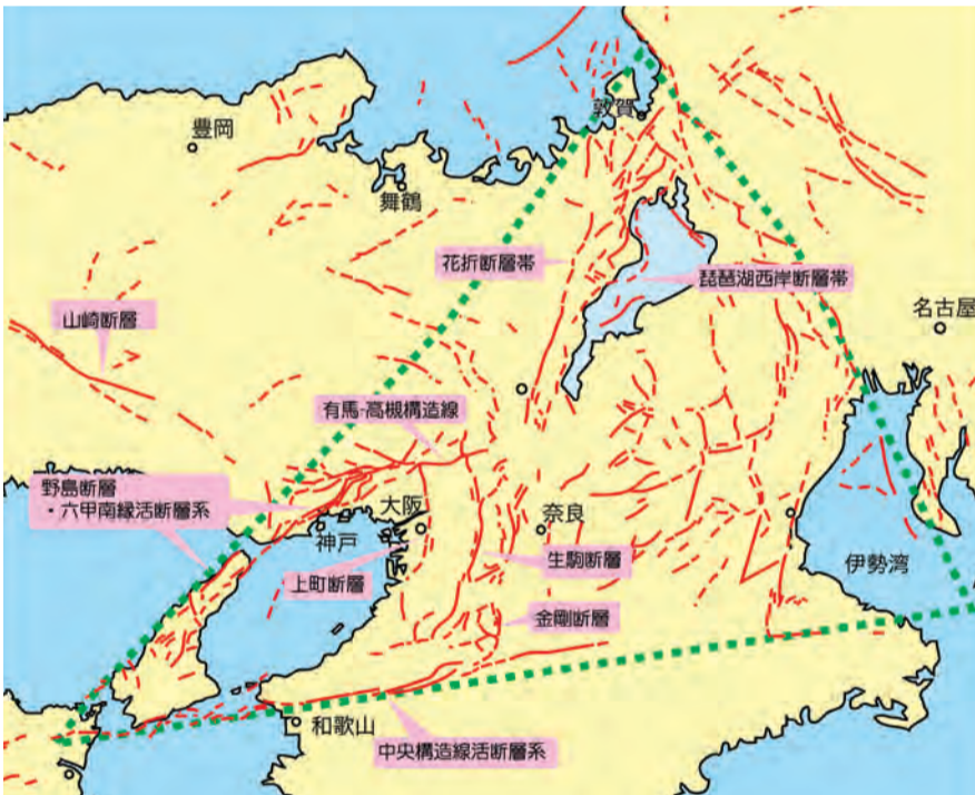
近畿地方周辺に見られる活断層の分布（活断層研究会、1991年『新編日本の活断層』に基づいて作成）。緑の点線が近畿トライアングル
