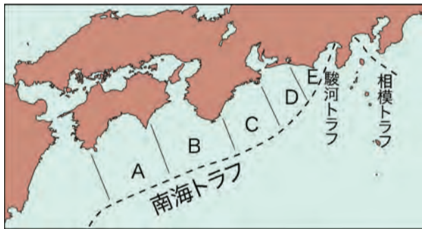
図：南海地震震源域
